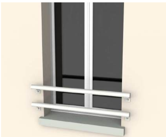
Barres d'appui posées en façade (allège minimum 600mm)
