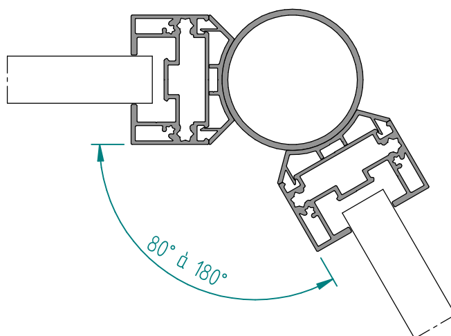
Poteau d'angle variable
